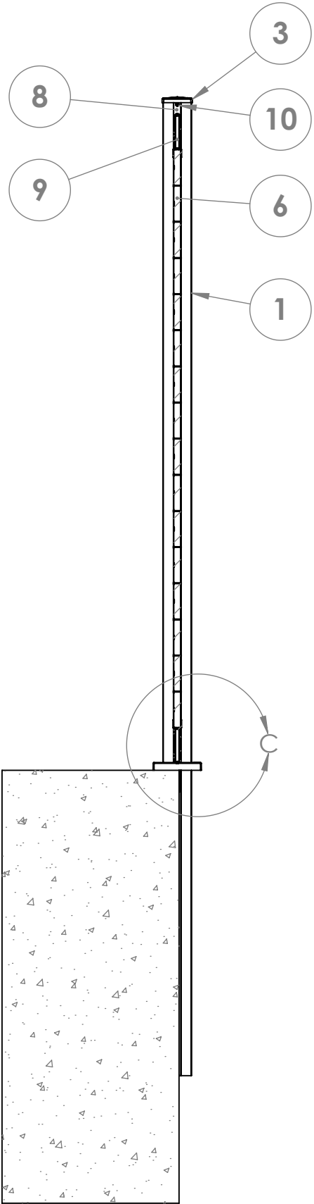
SECTION A-A SCALE 1 : 15
