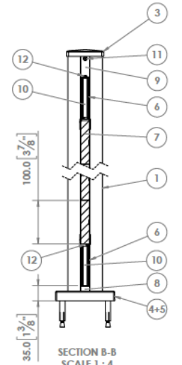
SECTION B-B SCALE 1 : 4
