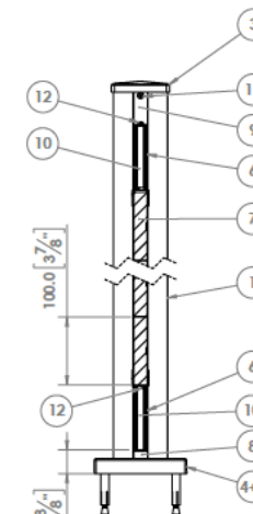
SECTION B-B SCALE 1 : 4
